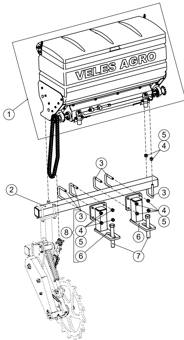
Бункер с приводом ГРС-4-01-02.000-05
