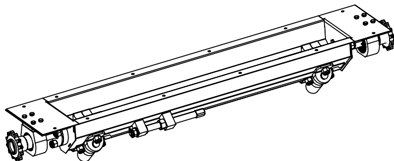
Лоток удобрений ГРС-4-09.500-09 в сборе
