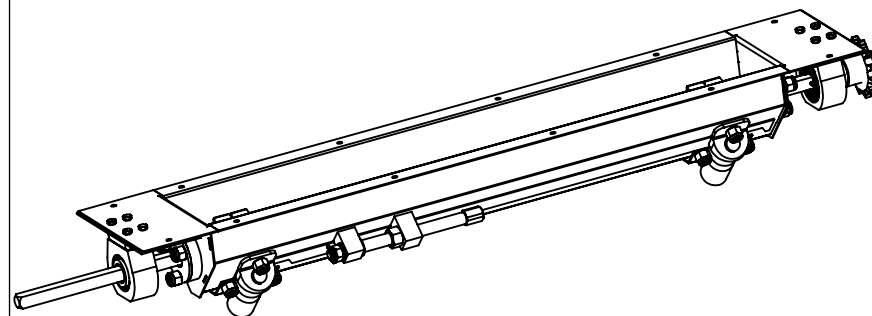
Лоток удобрений ГРС-4-09.500-10 в сборе
