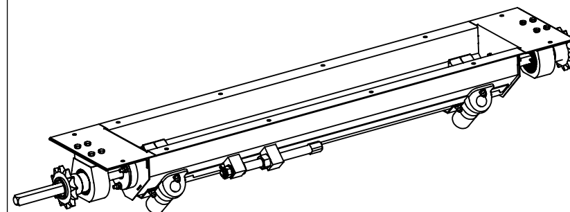
Лоток удобрений ГРС-4-09.500-04 в сборе
