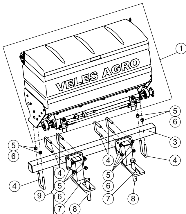
Бункер с приводом ГРС-4-01-02.000-04
