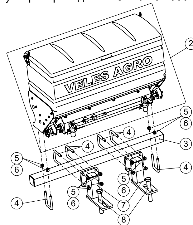
Бункер с приводом ГРС-4-01-02.000-03
