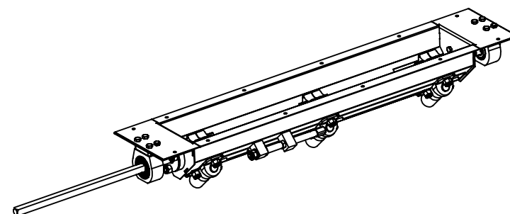
Лоток удобрений ГРС-4-09.500-02 в сборе
