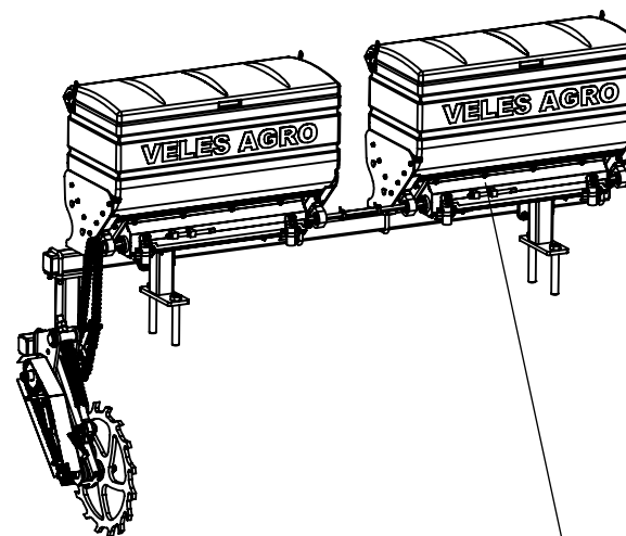
Лоток удобрений ГРС-4-09.500-02 в сборе
